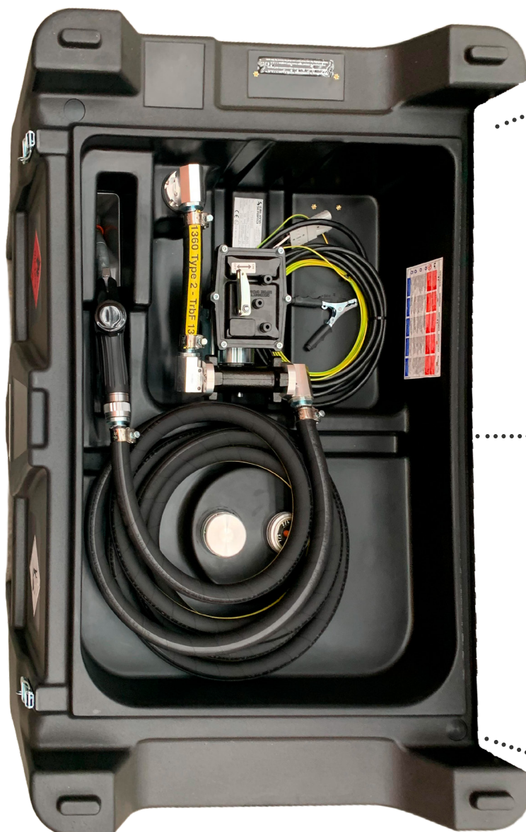
CABLE ELÉCTRICO Y PINZAS PARA CONEXIÓN A BATERIA
